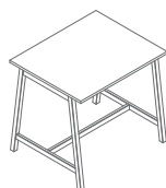
PSM722 1215 / 1000 / 1100 54 kg
