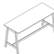
PSM88 1815 / 700 / 900 57.55 kg
