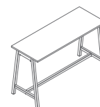
PSM78 1815 / 700 / 1100 60.05 kg
