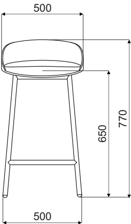
TE11H TE11HF
